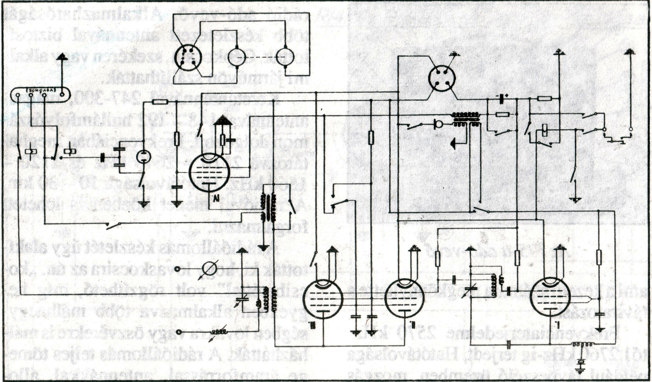
Az R/7-a adó elvi kapcsolása
