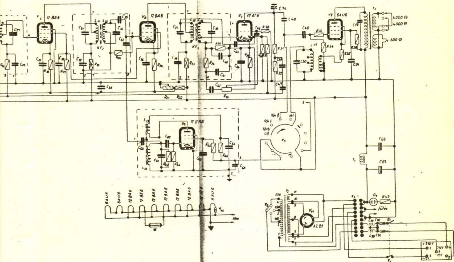
vevőkészülék részletes elvi kapcsolási vázlata
